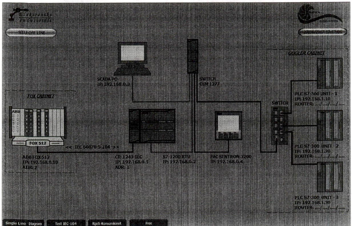
Fig.3. Arkitektura e paisjeve dhe rrjeti i komunikimit, nese shfaqen probleme ne komunikim atehere pervecse gjendjes se alarmit do te shfaqet dhe nderpreja e lidhjes me ngjyre te kuqe, ne te kundert ajo eshte e gjelber.
